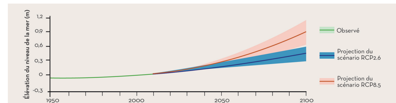
Figure 2 : Élévation globale du niveau moyen de la mer de 1950 à 2100, comparée à la période 1986-2005.
