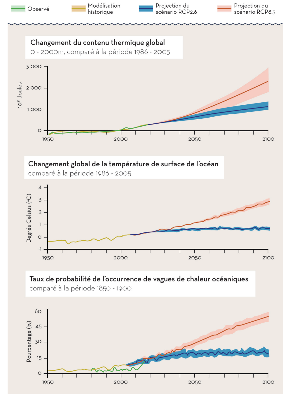
Figure 2 : Changements affectant l'océan : observations et projections concernant le contenu thermique et la probabilité de l'occurrence de vagues de chaleur selon les scénarios d'émissions basses (RCP2.6) et hautes (RCP8.5). Source: IPCC, SROCC, 2019. SPM
