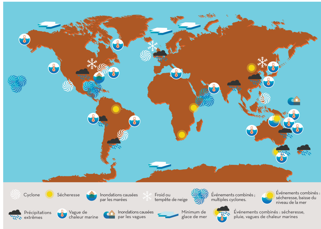
Figure 2 : Localisations des régions où se sont produits les événements extrêmes en lien avec les changements affectant l'océan (sélection d'événements qui ont eu lieu entre 1998 et 2017).
